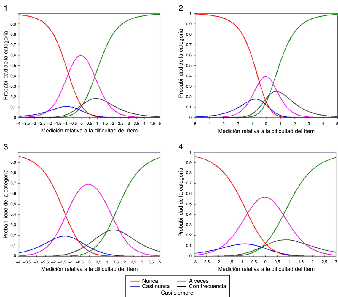
Figura 3 – Curvas características del ítem para la versión de niños. Dimensiones emocional (1), física (2), escolar (3) y social (4). El eje y señala la probabilidad de responder a cada categoría de respuesta (0-1). El eje x señala la dificultad del ítem medido en unidades logarítmicas, donde 0 representa la dificultad promedio; los valores negativos, menor dificultad y los valores positivos, mayor dificultad. Cuando menor es la dificultad del ítem (se aleja de 0 hacia valores negativos), la probabilidad de contestar «nunca» se acerca a 1 y la de contestar «casi siempre» es o se aproxima a 0. Nótese que cuando la dificultad del ítem está alrededor de 0, los umbrales se hacen desordenados y es más difícil separar patrones de respuesta.
