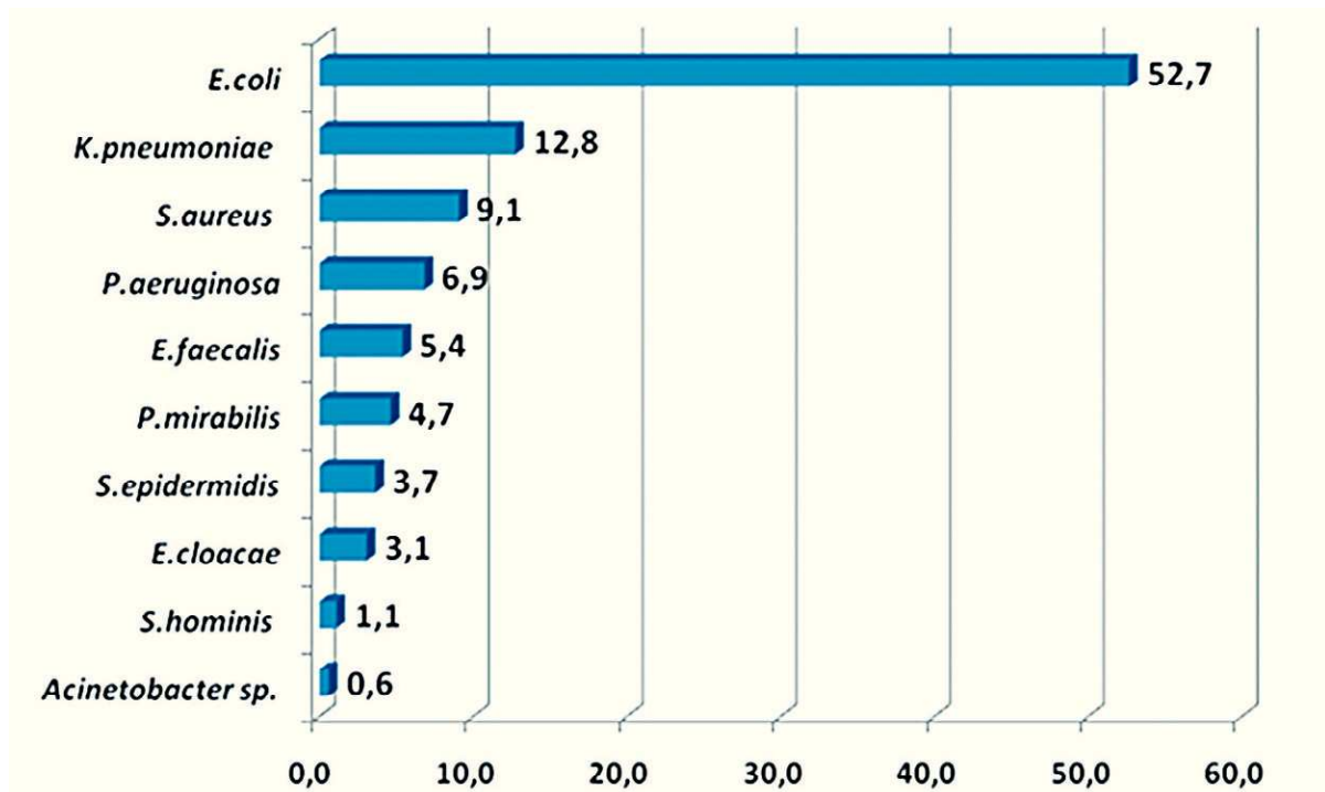
Figura 1 Distribución de los 10 aislamientos microbiológicos prevalentes. RENOVA 2010-2012 (n = 111.036).
