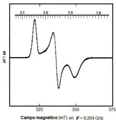
Figura 8. Espectros de RPE de ferredoxina reducida [2Fe-2S] de Synechococcus (Hearshen et al. , 1986).
