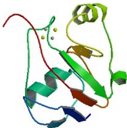
Figura 2. Estructura cristalina de ferredoxina [2Fe-2S] de Escherichia coli , tipo adrenoxina, PDB 1I7H.
