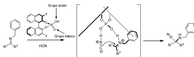
Figura 4. Modelo de la activación de iminas proquirales mediante un ácido fosfórico bifuncional.
