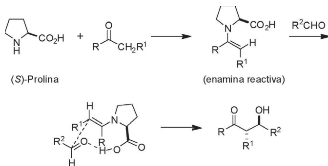
Figura 2. Activación de compuestos carbonílicos mediante ( S )-prolina.
