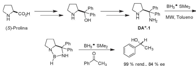
Figura 3. Síntesis y aplicación de la difenilprolinilamina DA*-1.
