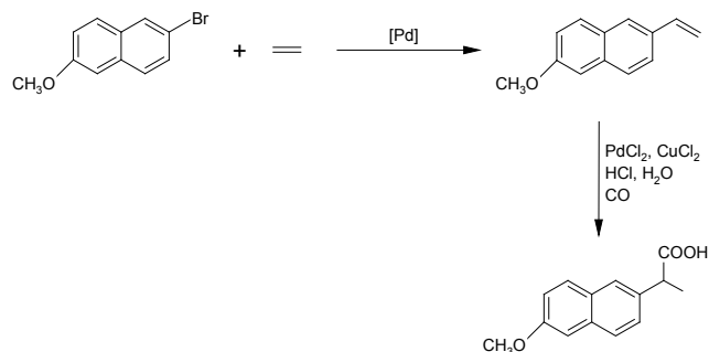
Figura 3. Síntesis de naproxeno
