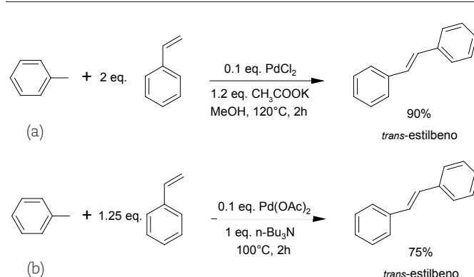
Figura 1. Reacciones informadas por (a) Mizoroki en 1971, y (b) Heck y Nolley en 1972.
