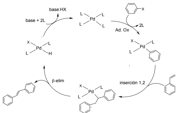
Figura 2. Mecanismo de la reacción de Heck.
