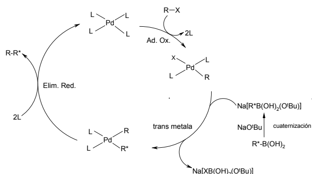
Figura 5. Mecanismo de la reacción de Suzuki.
