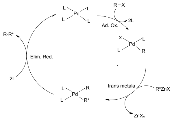
Figura 4. Mecanismo de la reacción de Negishi.
