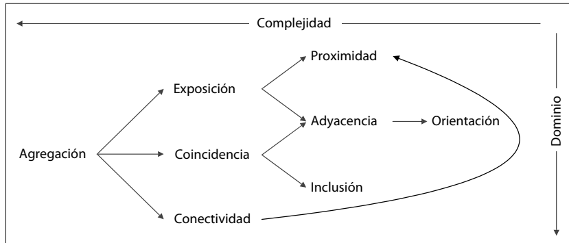
Figura 6. Dependencia espacial.
