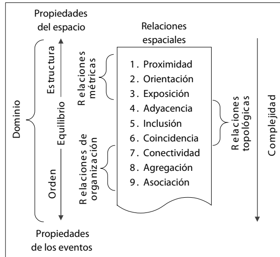
Figura 1. Relaciones espaciales.
