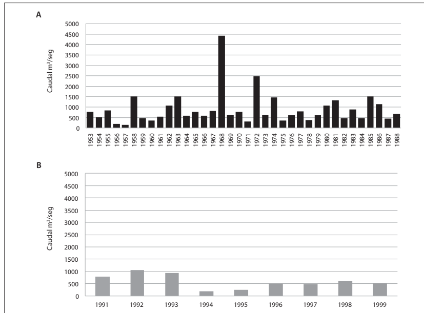
Figura 5. Caudal máxim anual de las series de 1953 a 1989 (A) y de 1990 a 1999 (B).
