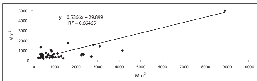
Figura 8. Correlación entre los caudales máximos diarios de las series de los ríos Acaponeta (eje X) y Piaxtla (eje Y).
