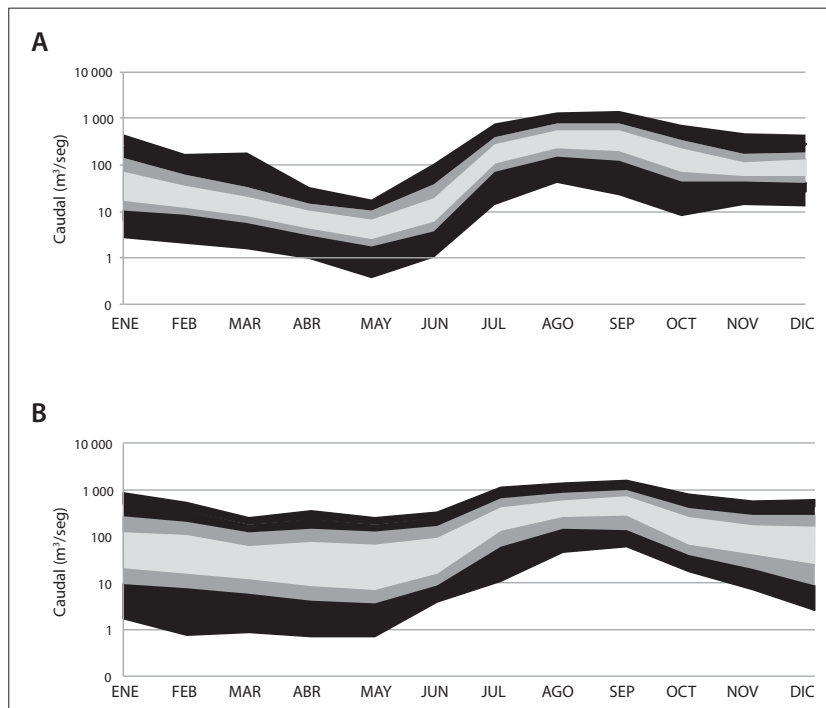
Figura 3. Patrones hidrológicos en régimen natural para el río Piactla (periodos: A 36 y B nueve años), los resultados están representados en escala logarítmica. Las diferentes tonalidades de gris muestran las probabilidades de ocurrencia de los caudales mensuales: negro intervalo entre el percentil 5-95; gris intervalo entre el percentil 10-90 y gris claro entre el percentil 25-75.
