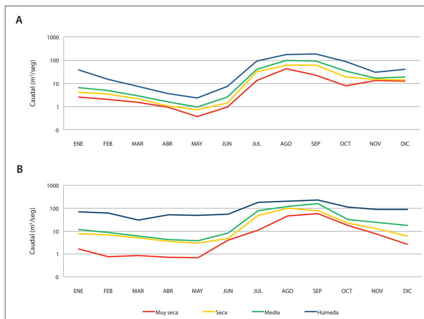
Figura 4. Régimen de caudales ordinarios estacionales para los periodos de A 36 y B nueve años.
