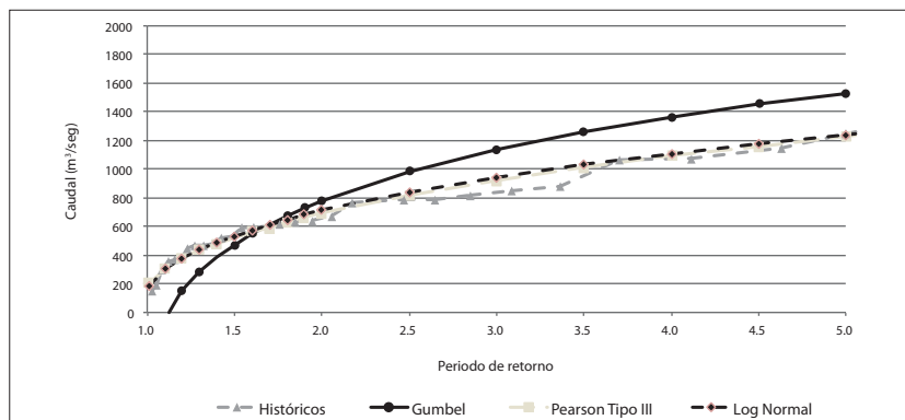
Figura 6. Distribución estadística para identificar la magnitud de las avenidas a distintos periodos de retorno del río Piaxtla.
