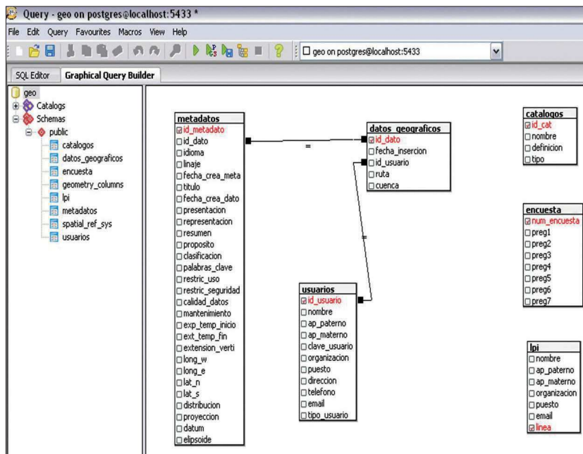
Figura 3. Modelo físico de la GeoBase-L9 en PostgreSQL.
