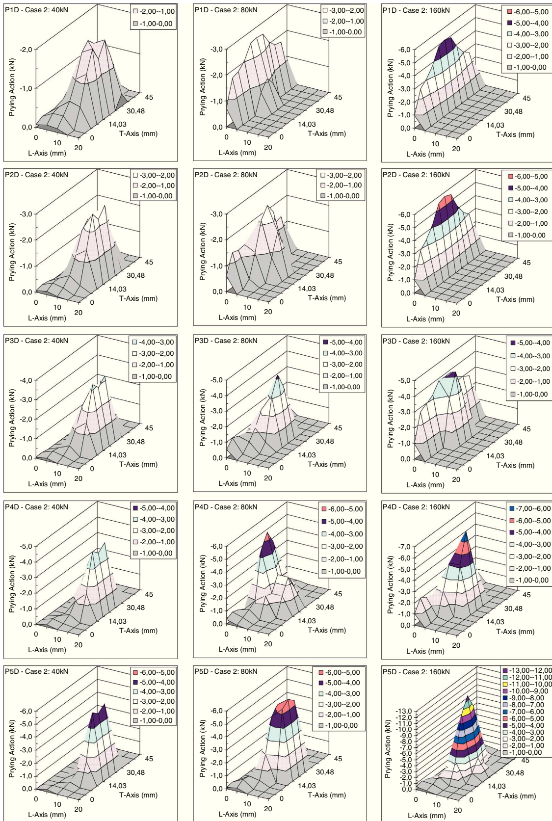
Figura 8. Distribución de la acción de apalancamiento para el caso 2 (precarga).
