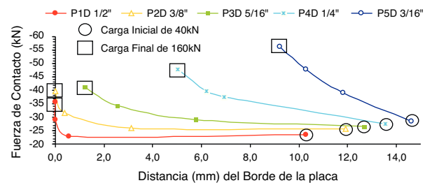
Figura 19. Resultante de fuerza de contacto y distancia al borde de la placa: caso 2.
