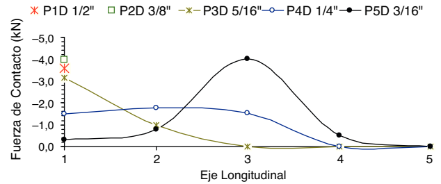
Figura 18. Fuerza de contacto a lo largo del eje L para 160 kN: caso 2.
