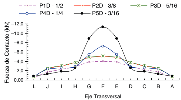
Figura 13. Fuerzas resultantes de contacto a lo largo del eje T-160 kN: caso 1.
