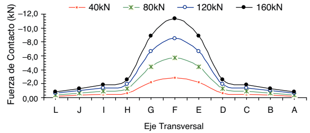
Figura 11. Resultante de las fuerzas a lo largo del eje transversal de P5D: caso 1.
