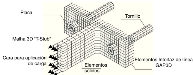
Figura 4. Malla completa del «T-Stub» para los modelos P1D, P2D, P3D, P4D y P5D.
