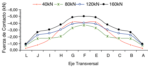
Figura 15. Resultante de la fuerza de contacto a lo largo del eje T para P1D: caso 2.
