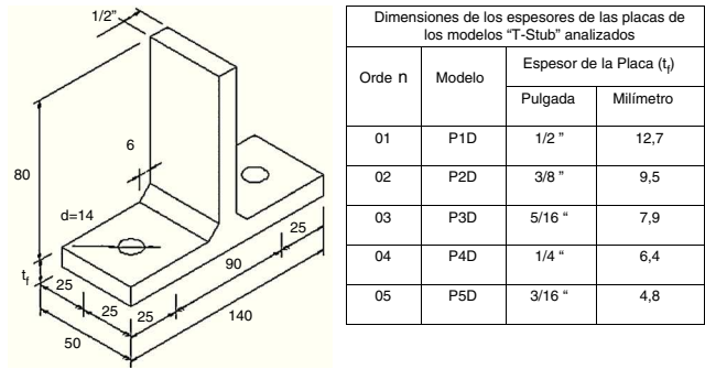
Figura 2. Dimensiones «T-Stub» (en milímetros).
