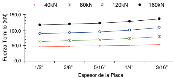
Figura 23. Relación de la fuerza en uno tornillo y el espesor de la placa: caso 2.
