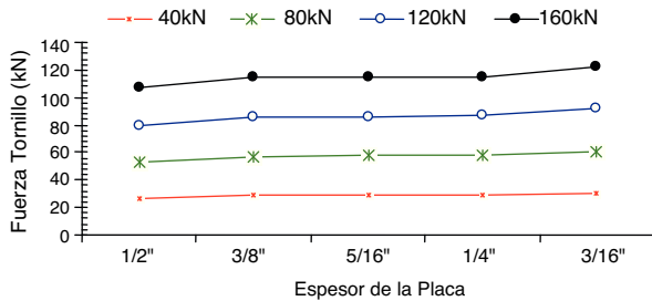
Figura 22. Relación de la fuerza en uno tornillo y el espesor de la placa: caso 1.
