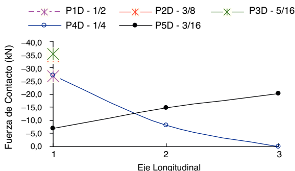
Figura 17. Fuerza de contacto a lo largo del eje L para 160 kN: caso 1.
