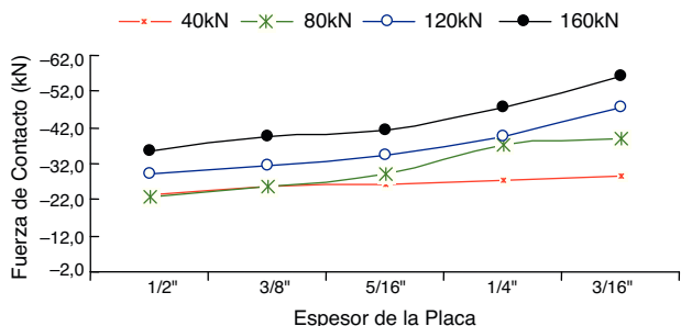
Figura 10. Variación de la resultante en función del espesor de la placa: caso 2.
