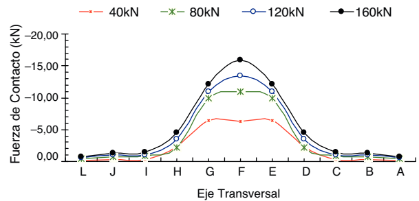
Figura 14. Fuerza resultante de contacto a lo largo del eje T para P5D: caso 2.
