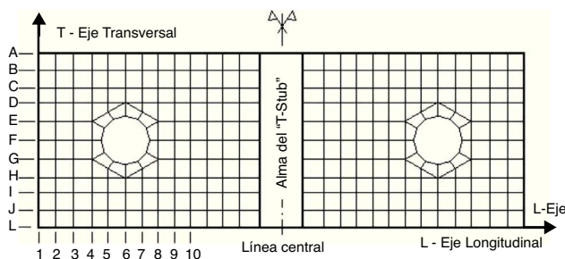
Figura 6. Identificación de ejes y nodos de la malla en la interfaz de contacto.
