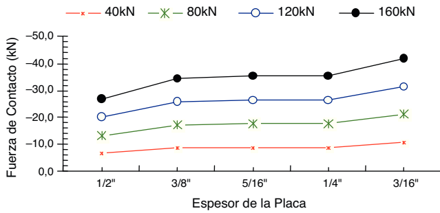
Figura 9. Variación de la resultante en función del espesor de la placa: caso 1.
