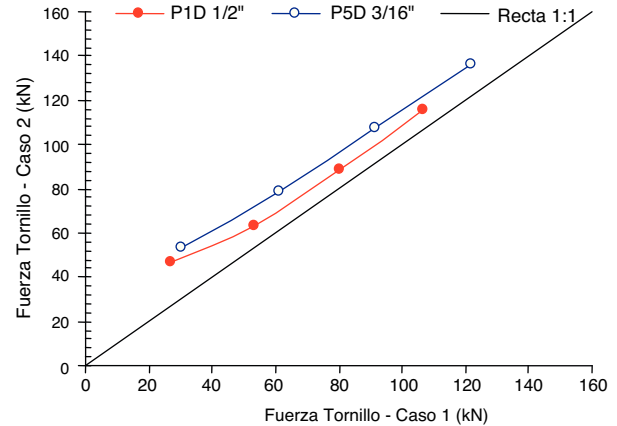
Figura 24. Relación entre la RFC en el caso 2 y el caso 1.
