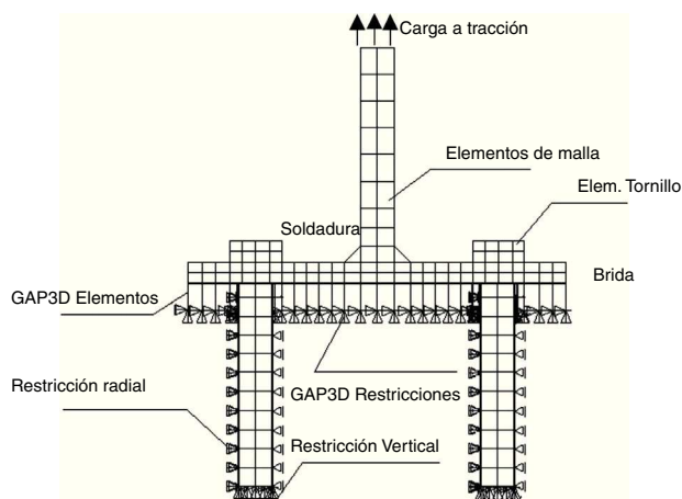
Figura 5. Malla de los elementos de la interfaz y del contorno.
