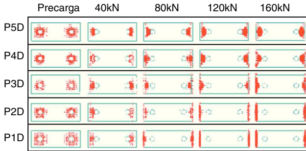
Figura 21. Evolución de la distribución de la fuerza de contacto para el caso 2.
