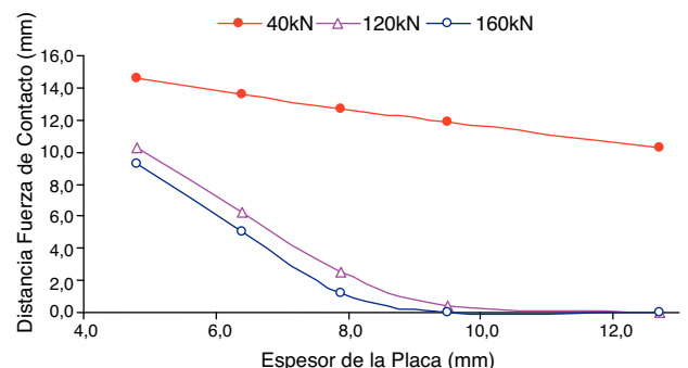
Figura 20. Distancia de las RFC hasta al borde vs espesor de la placa: caso 2.
