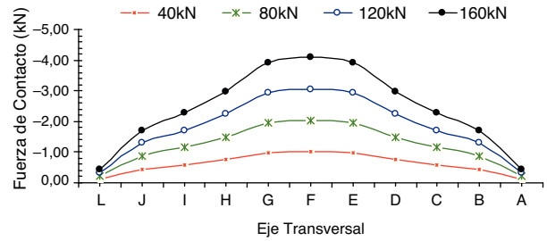
Figura 12. Fuerzas resultantes de contacto a lo largo del eje T para P1D: caso 1.
