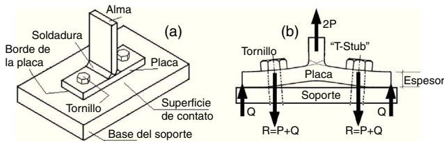
Figura 1. a) Conexión de acero «T-Stub». b) Modelo analítico usual.
