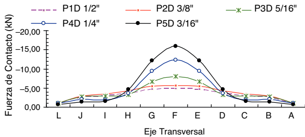
Figura 16. Resultante de la fuerza de contacto a lo largo del eje T para 160 kN: caso 2.
