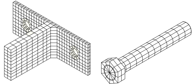
Figura 3. Mallas de EF para la conexión «T-Stub» con los tornillos.
