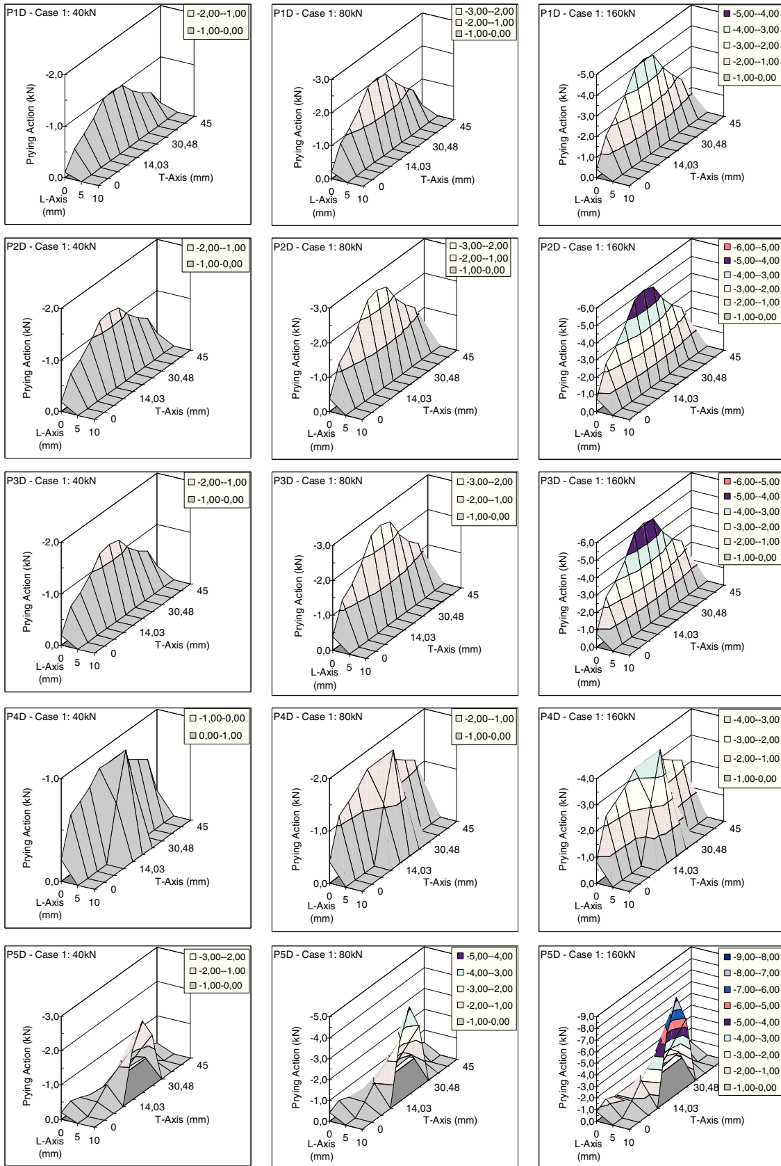
Figura 7. Distribución de la acción de apalancamiento para el caso 1 (sin precarga).
