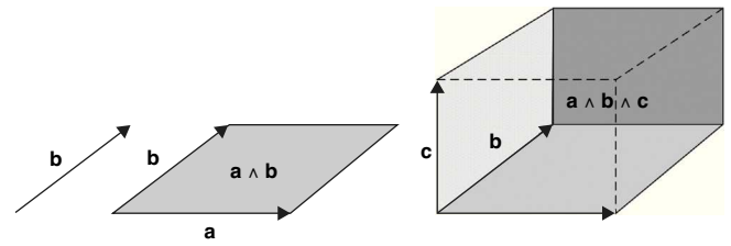
Figura 1. Objetos geométricos.
