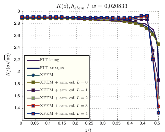
Figura 8. FIT, tamaño de elemento inferior a la región afectada, h_{elem}=0,062a .
