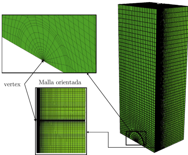
Figura 4. Malla adaptada al problema en ABAQUS. Se puede observar el refinamiento concentrado hacia el vertex.
