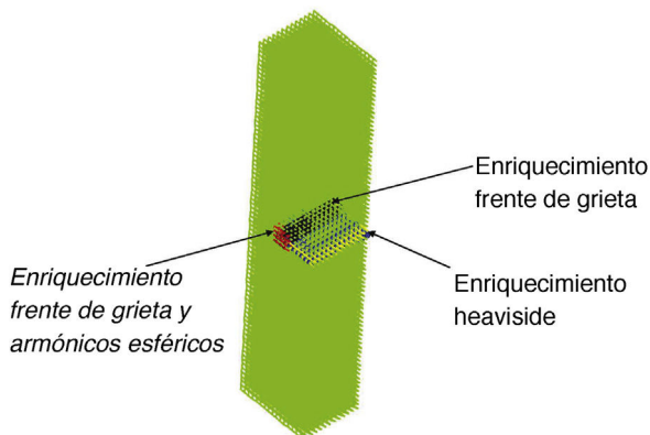
Figura 5. Ejemplo de una de las mallas para el análisis con XFEM. Se pueden observar las regiones enriquecidas.
