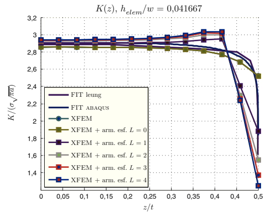
Figura 6. FIT, tamaño de elemento mayor que la región afectada, h_{elem}=0,125a .
