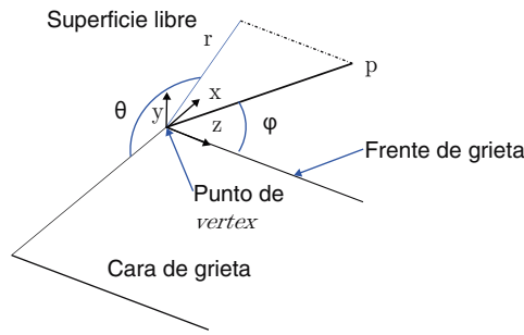
Figura 1. Sistema esférico de coordenadas definido en el punto de intersección de la grieta con la superficie libre.
