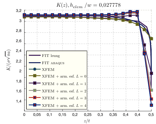
Figura 7. FIT, tamaño de elemento similar a la región afectada, h_{elem}=0,083a .
