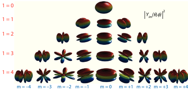
Figura 2. Ilustración que muestra la forma de los primeros armónicos esféricos l=0, 1, 2, 3, 4 .
