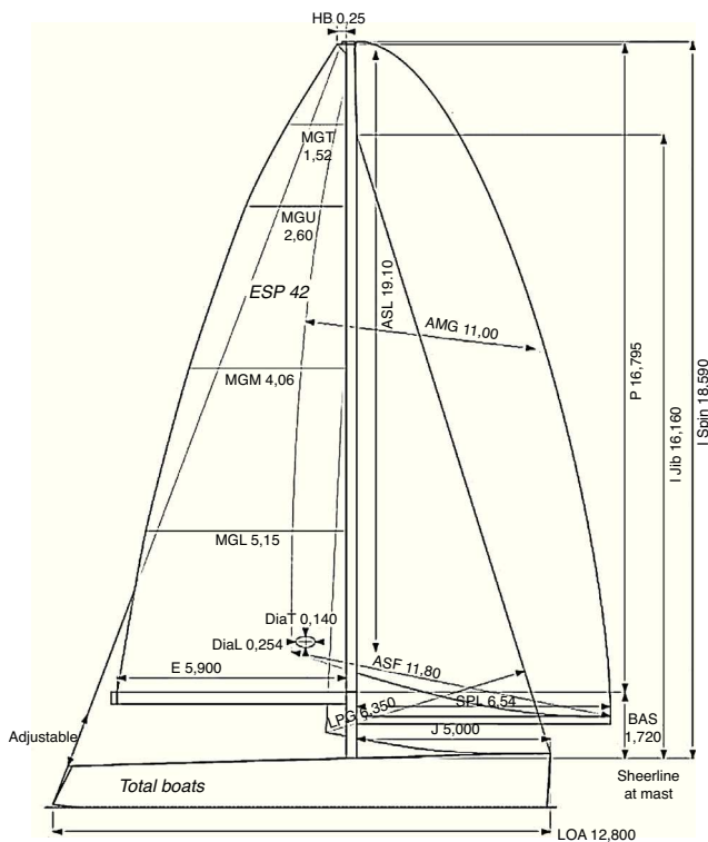
Figura 10. Plano vélico del velero Totalboats GP42.
