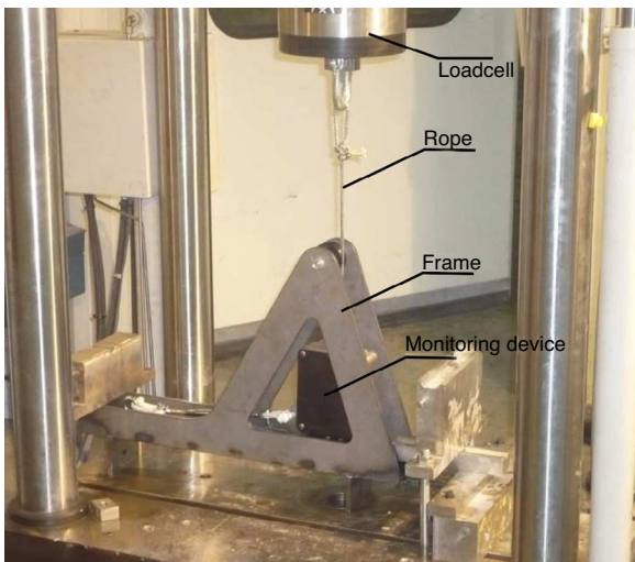
Figura 4. Disposición experimental del prototipo del arraigo.
