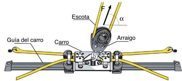
Figura 2. Esquema de un carro de mayor típico.
