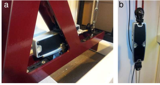
Figura 9. Desarrollo de los experimentos del 3D Remote Rigging Monitor (modos de configuración de la fuerza y el ángulo, a la izquierda, y de carga, a la derecha).
