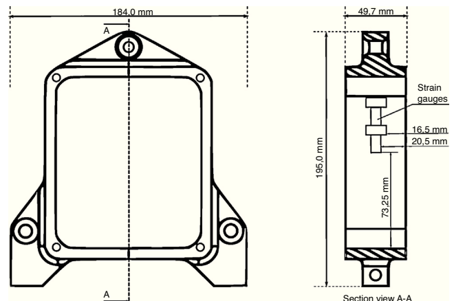
Figura 3. Plano del prototipo de arraigo sensorizado.
