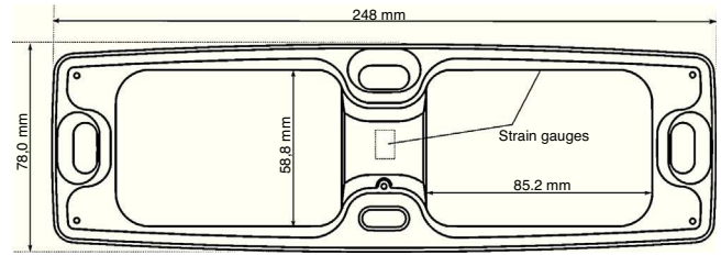
Figura 7. Diseño del 3D Remote Rigging Monitor.
