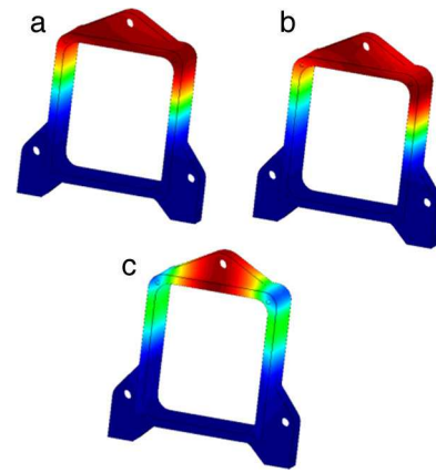
Figura 6. Resultados del campo de desplazamientos en el modelo FEM. De izquierda a derecha: carga 4,5 kN-29°, 2,25 kN-13° y 2,25 kN-0°.
