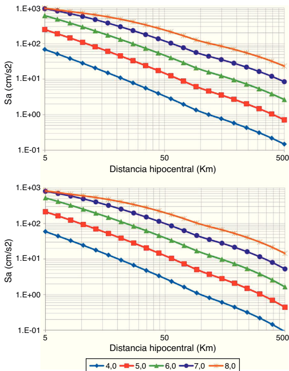
Figura 5. Relaciones de atenuación de movimiento fuerte utilizadas para PGA: zona intraplaca (a la izquierda) y zona de subducción (a la derecha). Magnitudes en M_w .
