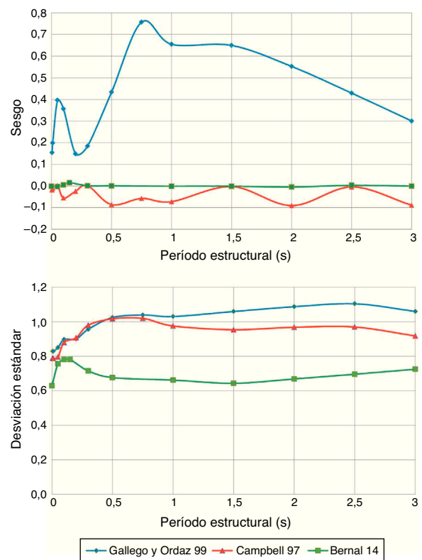
Figura 6. Comparación de sesgos (a la izquierda) y desviaciones estándar (a la derecha) entre diferentes modelos de atenuación de movimiento fuerte para sismos intraplaca.
