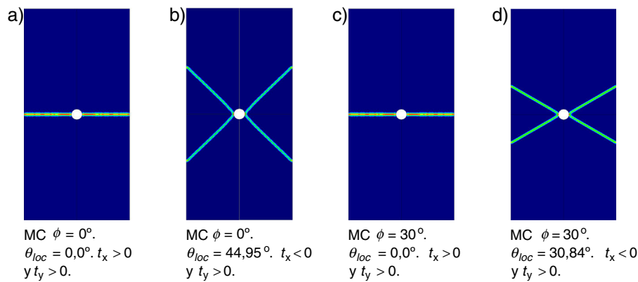
Figura 10. Deformación plástica equivalente para diferentes valores de \phi en modelo MC en tensión plana.
