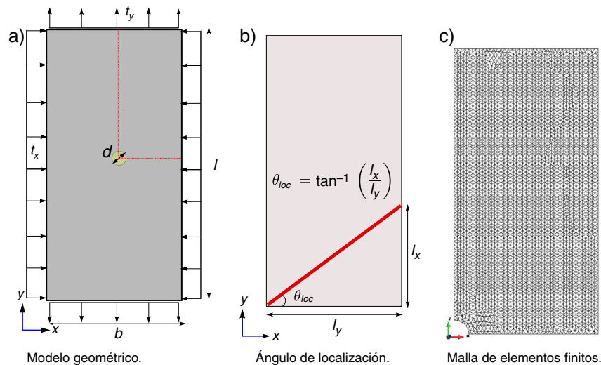
Figura 7. Geometría y malla empleada.
