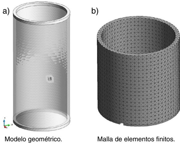
Figura 12. Geometría y malla empleada.
