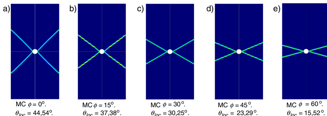
Figura 8. Deformación plástica equivalente para diferentes valores de \phi en modelo MC en deformación plana.
