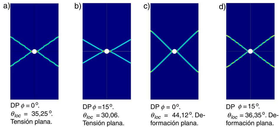
Figura 9. Deformación plástica equivalente para diferentes valores de \phi en modelo DP.
