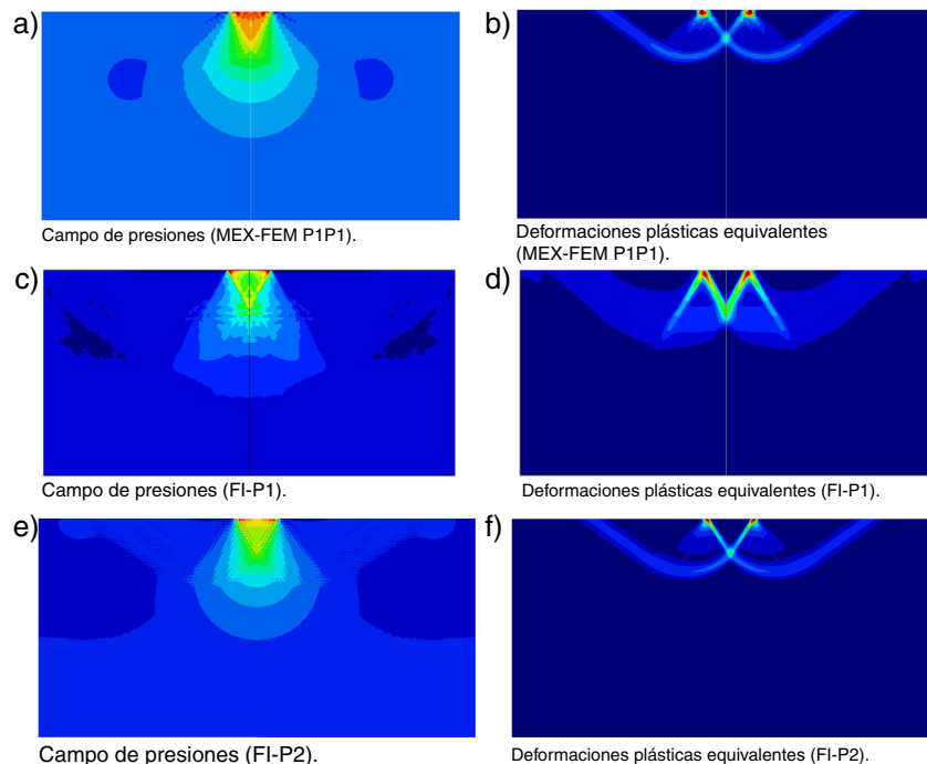
Figura 5. Comparación de los campos de presión y deformación plástica equivalente obtenidas con MEX-FEM y formulación estándar en desplazamientos.
