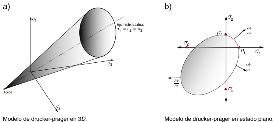
Figura 2. Modelo de Drucker-Prager.
