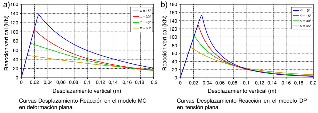
Figura 11. Curvas Desplazamiento-Reacción.
