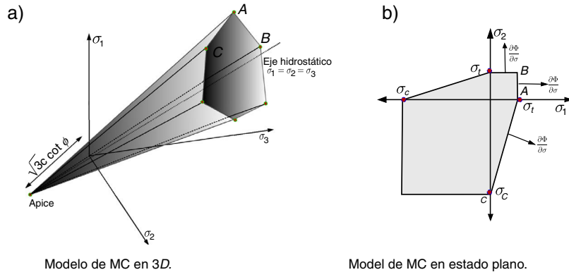
Figura 1. Modelo de Mohr-Coulomb.
