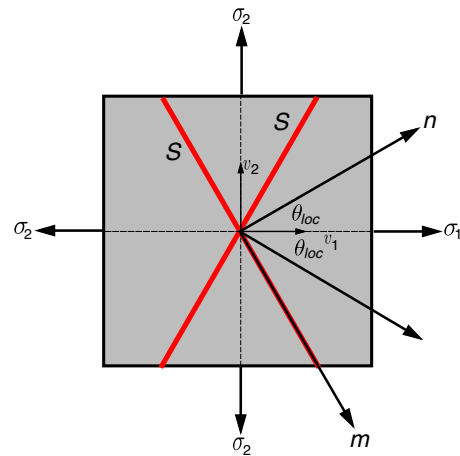
Figura 3. Ángulo de localización.
