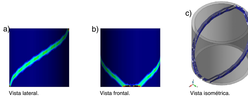
Figura 13. Deformaciones plásticas equivalentes en el modelo de VM en tracción pura. Ángulo de localización teórico: \theta_{loc}^{teo} = \pm 45.0^\circ con el eje vertical. Ángulo de localización numérico: \theta_{loc}^{num} = \pm 45.0^\circ .
