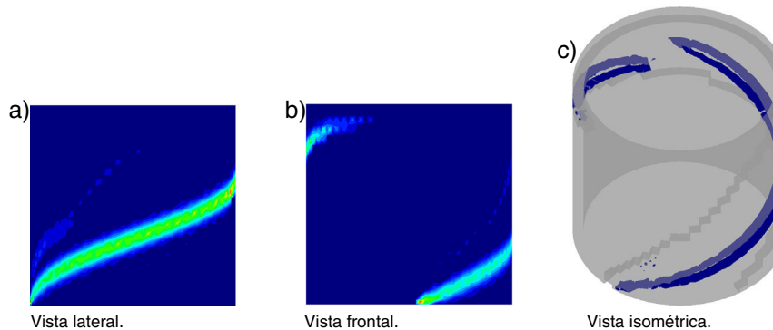
Figura 14. Deformaciones plásticas equivalentes en el modelo de MC con \phi = 45^\circ en torsión con perturbación de tracción. Ángulo de localización teórico: \theta_{loc}^{teo} = 22.5^\circ con el plano horizontal. Ángulo de localización numérico: \theta_{loc}^{num} = 23.62^\circ .
