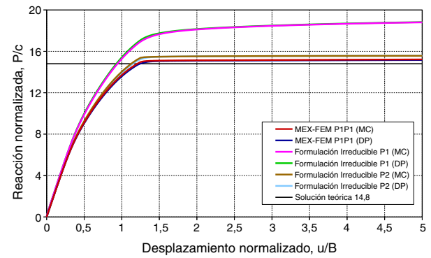
Figura 6. Curva Desplazamiento-Reacción.
