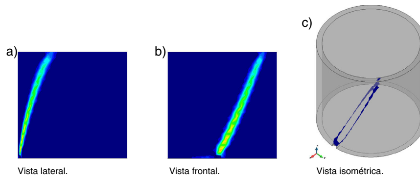
Figura 15. Deformaciones plásticas equivalentes en el modelo de MC con \phi = 45^\circ en torsión pura. Ángulo de localización teórico: \theta_{loc}^{teo} = 67.5^\circ con el plano horizontal. Ángulo de localización numérico: \theta_{loc}^{num} = 67.53^\circ .
