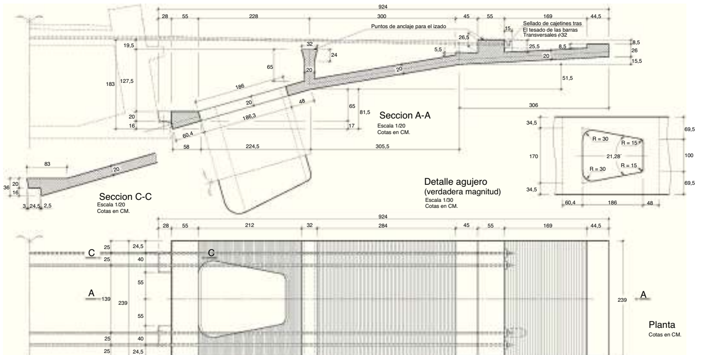
Figura 7. Definición de las piezas prefabricadas de voladizos.
