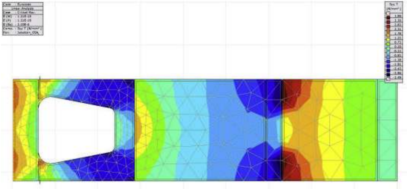
Figura 9. Vista del modelo de cálculo de detalle de jabalcones.
