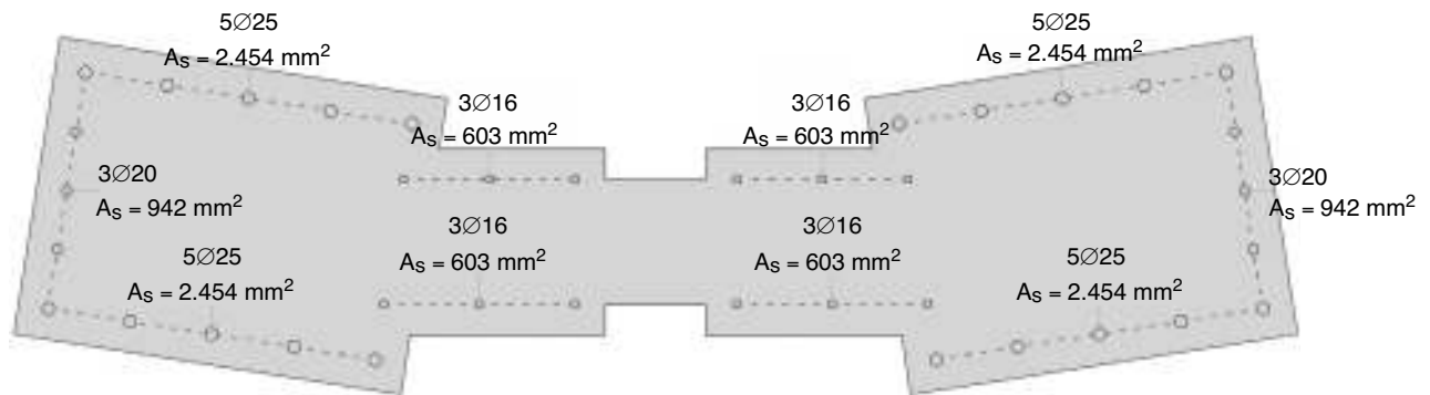
Figura 10. Sección de cálculo en clave del arco.
