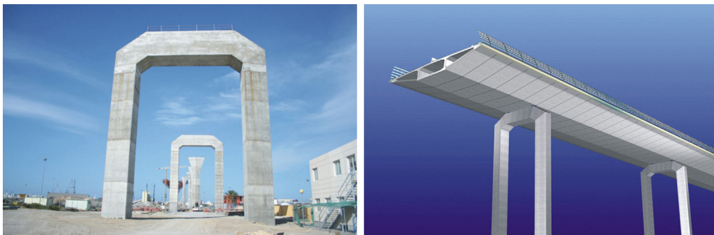
Figura 30. Pilas dobles por presencia de calzada bajo el tablero.
