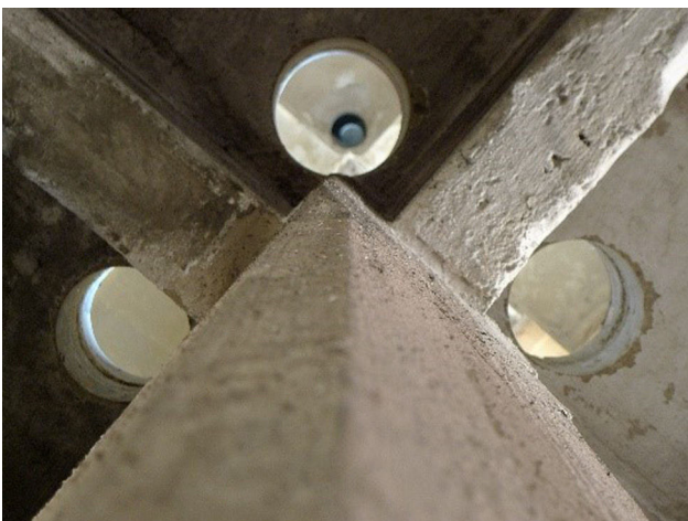
Figura 5. Huevo para paso de los nuevos pilares a través de las losas existentes.
