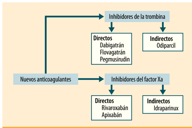
Figura 1. Nuevos anticoagulantes
