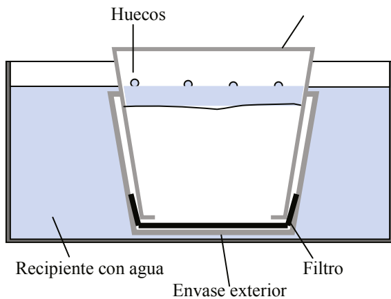
Figura 6. Gráfico del ensayo de absorción modificado Fuente: Henneberg de León (2010)
