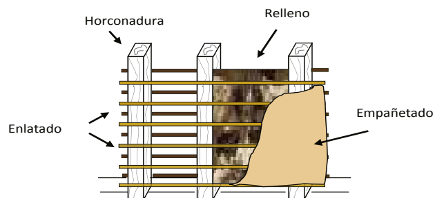
Figura 1. Componentes del bahareque (Henneberg de León, 2012)
