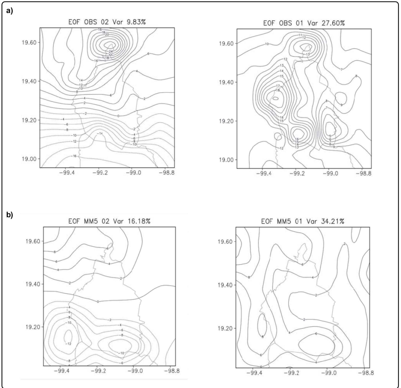
Figura 4. Modos de variabilidad EOFs para (a) observaciones y (b) modelo de mesoescala MM5.
