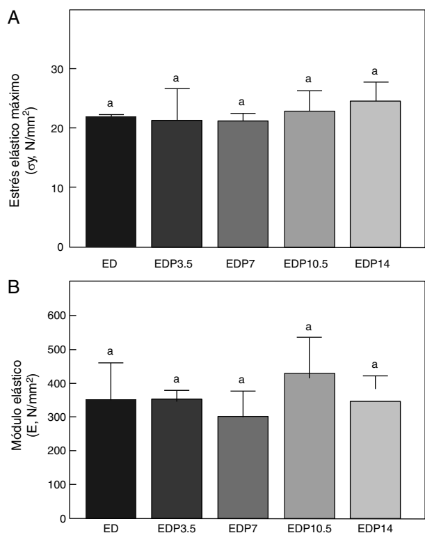
Figura 8 Propiedades materiales. A: estrés elástico máximo ( \sigma_y ) y B: módulo elástico (E), del fémur de animales experimentales ED + propranolol 3,5 mg/kg/día (EDP3,5); experimentales ED + propranolol 7 mg/kg/día (EDP7); experimentales ED + propranolol 10,5 mg/kg/día (EDP10,5); experimentales ED + propranolol 14 mg/kg/día (EDP14) expresadas como porcentaje de incremento de dichas variables respecto de las correspondientes a ED a tiempo final (T4). Letras diferentes indican diferencias significativas entre grupos, donde ED = a ( p < 0,05 ).
