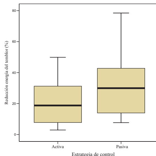
Figura 10. Comparación de los resultados obtenidos con cada una de las estrategias de control.
