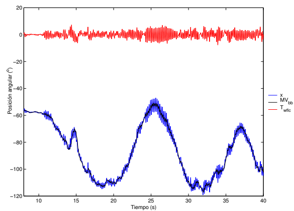
Figura 8. Ilustración del funcionamiento del algoritmo propuesto para la estimación del movimiento voluntario y del movimiento tembloroso con un retardo mínimo. El movimiento ( x ) corresponde a la articulación del codo de un paciente de temblor esencial al realizar la tarea de dibujar una espiral. El algoritmo está compuesto por dos etapas, en la primera se estima el movimiento voluntario mediante la utilización del filtro de Benedict-Bordner ( MV_{bb} ) y en la segunda etapa se estima el movimiento tembloroso ( T_{wflc} ) a través del WFLC.
