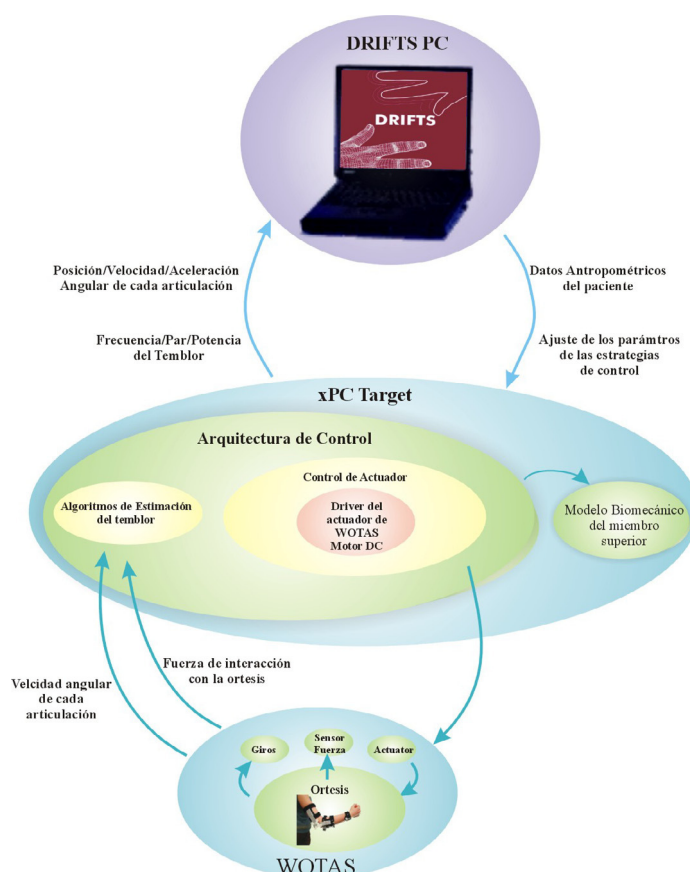
Figura 4. Arquitectura de control del exoesqueleto WOTAS.
