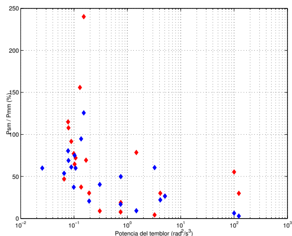
Figura 9. Relación entre la potencia espectral del movimiento tembloroso del paciente con WOTAS operando en modo de monitorización , P_{mm} , y la potencia espectral del movimiento tembloroso del paciente con WOTAS operando en los dos modos de supresión del temblor P_{ms} : modo activo - azul y modo pasivo - rojo. Esta relación cuantifica la reducción en la amplitud del temblor con la aplicación de las estrategias de control.
