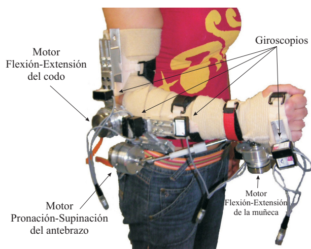
Figura 3. Versión final de WOTAS para el control de tres movimientos del miembro superior humano: flexión-extensión del codo, flexión-extensión de la muñeca y pronación-supinación del antebrazo.
