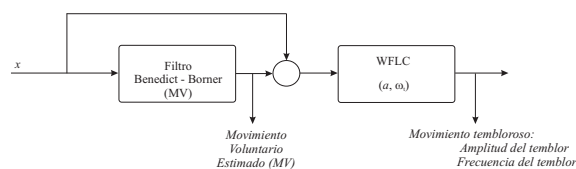
Figura 7. Algoritmo de dos etapas para la estimación del temblor y del movimiento tembloroso. En la primera etapa, se estima la amplitud del movimiento voluntario (MV) del movimiento total, x , mediante la utilización de un filtro de Benedict-Bordner. En la segunda etapa, el movimiento voluntario estimado en la primera etapa es removido de la señal de entrada y se asume que la señal restante es temblor. En esta etapa, se adopta el WFLC para la estimación tanto de la amplitud, a , como de la frecuencia del movimiento tembloroso, \omega_t .
