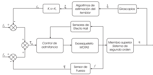
Figura 5. Estrategia de control para la modificación de la impedancia del miembro superior implementada en cada articulación del exoesqueleto WOTAS.
