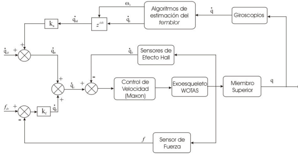
Figura 6. Estrategia de control repetitivo de velocidad implementada en el exoesqueleto WOTAS.
