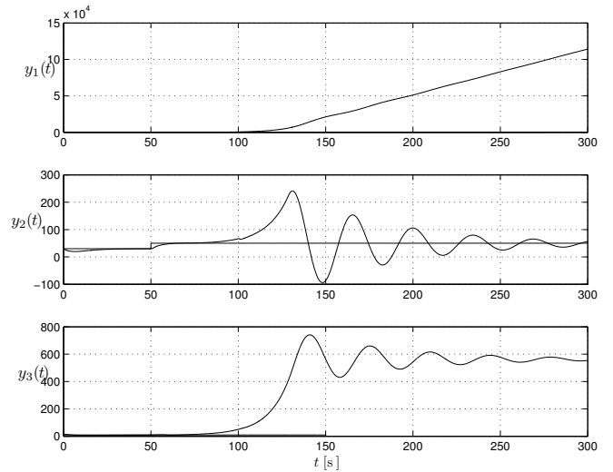
Figura 4. Salidas del sistema, saturado sin compensación.
