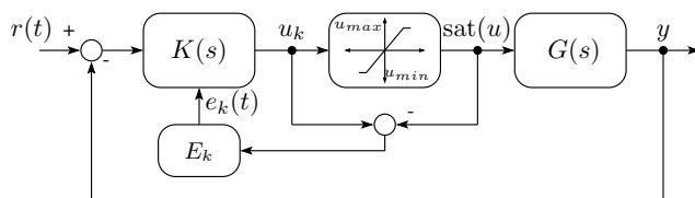
Figura 1. Compensación anti-windup.
