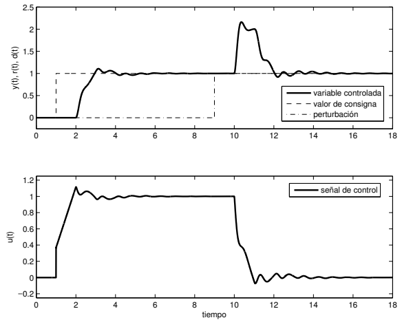
Figura 7. Comportamiento sistema de control, Planta 5
