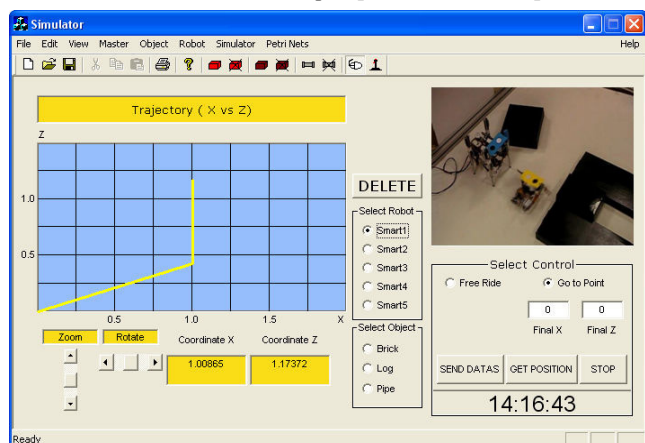
Figura 23: Aspecto de la Interfaz visual durante la tarea de cooperación.
