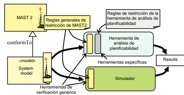
Figura 3. Ejemplo de modelos que requieren validación.
