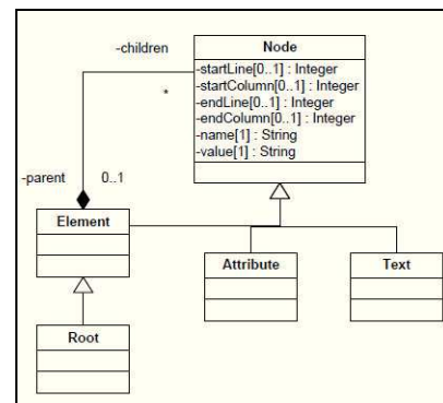
Figura 10. El meta-modelo XML
