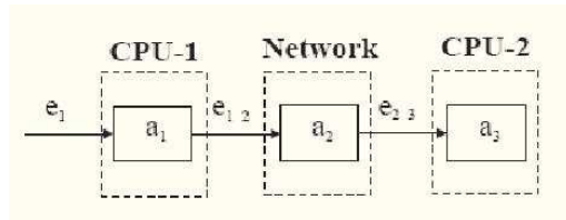
Figura 1: Modelo lineal
