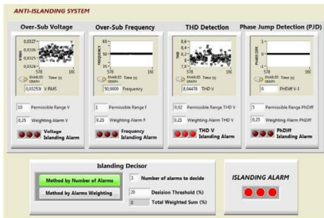
Figura 12: Pantalla de operación anti-islanding.
