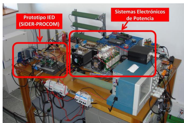
Figura 24: Escenario experimental para el inversor inteligente SIDER.
