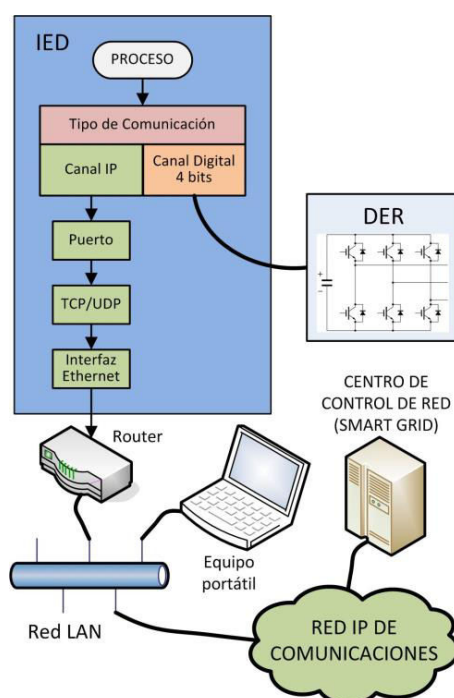
Figura 5: Funcionalidad de comunicaciones del IED.
