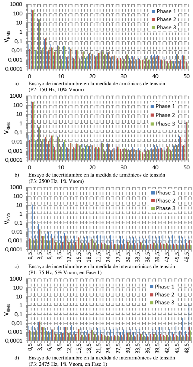
Figura 18: Espectros armónicos e interarmónicos de tensión registrados en las pruebas de clase A.
