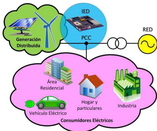
Figura 1: Contexto de aplicación del IED como control de la interconexión entre DER y el resto del sistema.
