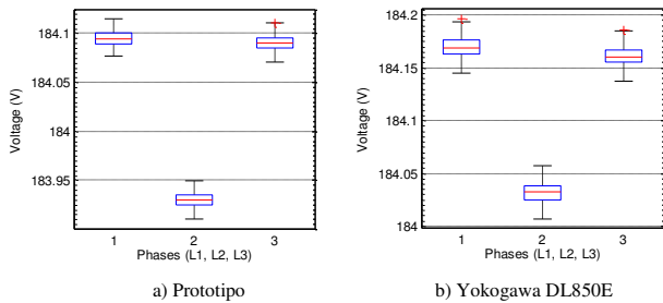
Figura 17: Comparación de medidas de tensión, en la prueba de clase A en P3 (80% V_{nom} ), entre el prototipo y el registrador Yokogawa DL850E.
