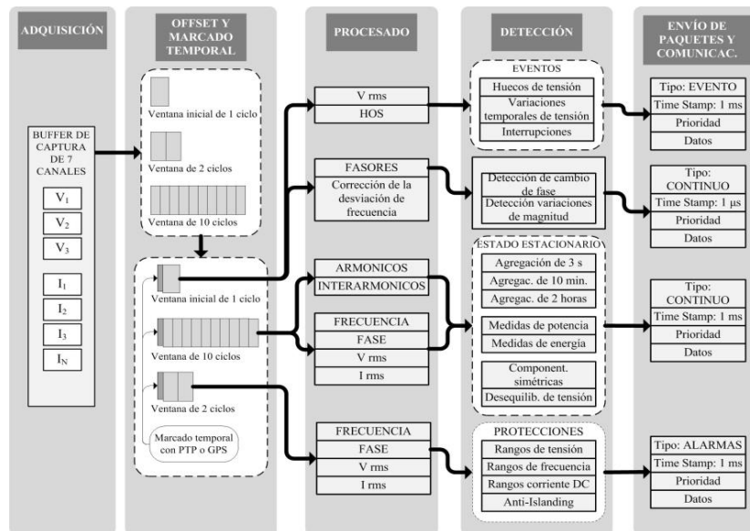
Figura 3: Etapas de la arquitectura funcional del IED desarrollado.
