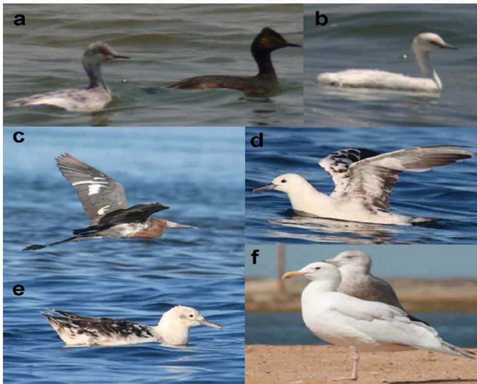
Figura 1. Aves acuáticas leucísticas observadas en el complejo de humedales de Guerrero Negro. a, b, P. nigricollis con diferentes grados de afectación de leucismo en sus plumas junto con un individuo de coloración normal; c, ave adulta de E. rufescens con leucismo; d, e, aves adultas de P. opisthomelas con diferentes niveles de afectación de leucismo, y f, individuo leucístico de L. occidentalis .
