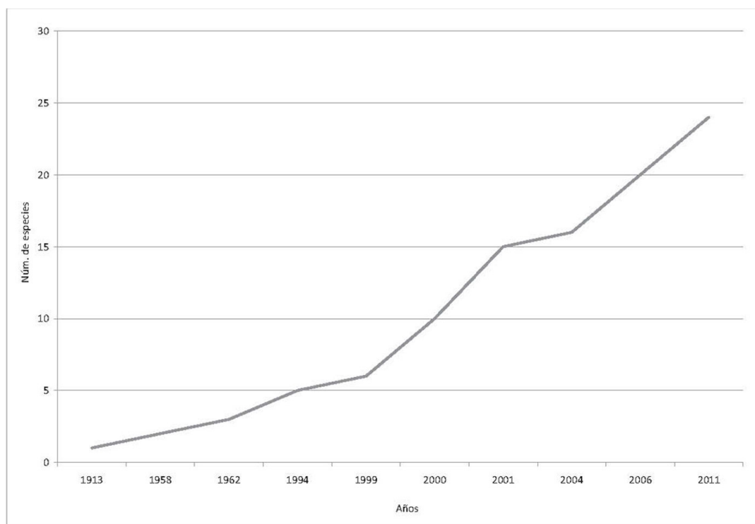
Figura 2. Curva acumulativa de especies descritas de Mecoptera (especies con holotipo de México).
