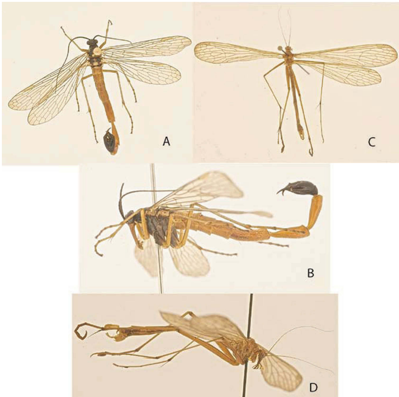
Figura 1. Hábito de Mecoptera. A), Panorpa sp. (macho), dorsal; B), Panorpa sp., macho, lateral; C), Bittacus sp. (macho), dorsal; D), Bittacus sp. (macho), lateral.
