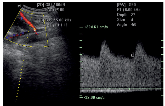
Figura 8: Forma de onda de velocidad de flujo de la arteria uterina en el primer trimestre. Se observa un notch protodiastólico (n) y escasa cantidad de flujo de fin de diástole (d) que definen a una forma de onda de elevada resistencia.
